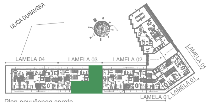
Plan povučenog sprata
